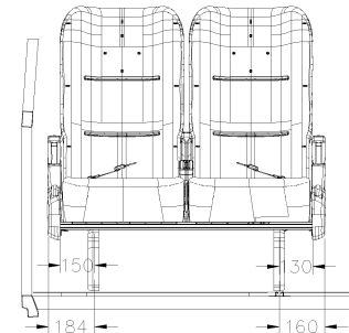
CROQUI MONTAGEM PE SOBRE PATAMAR
